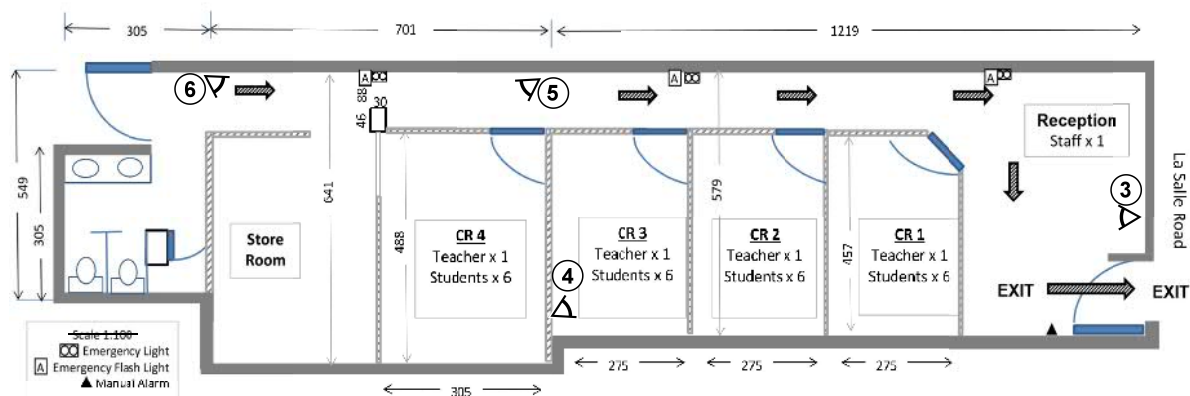
地下平面圖 GROUND FLOOR PLAN
