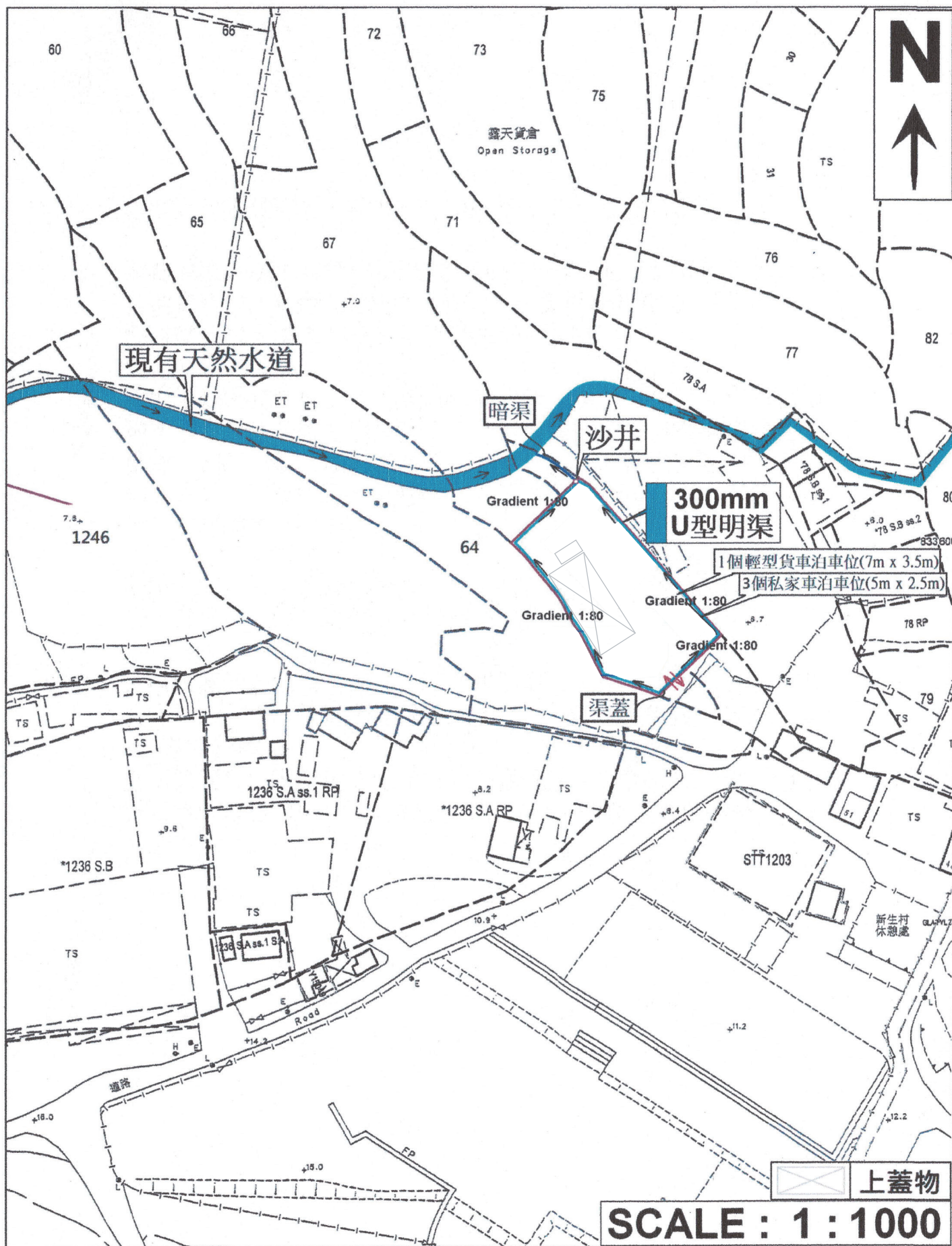
渠務建議計劃圖
