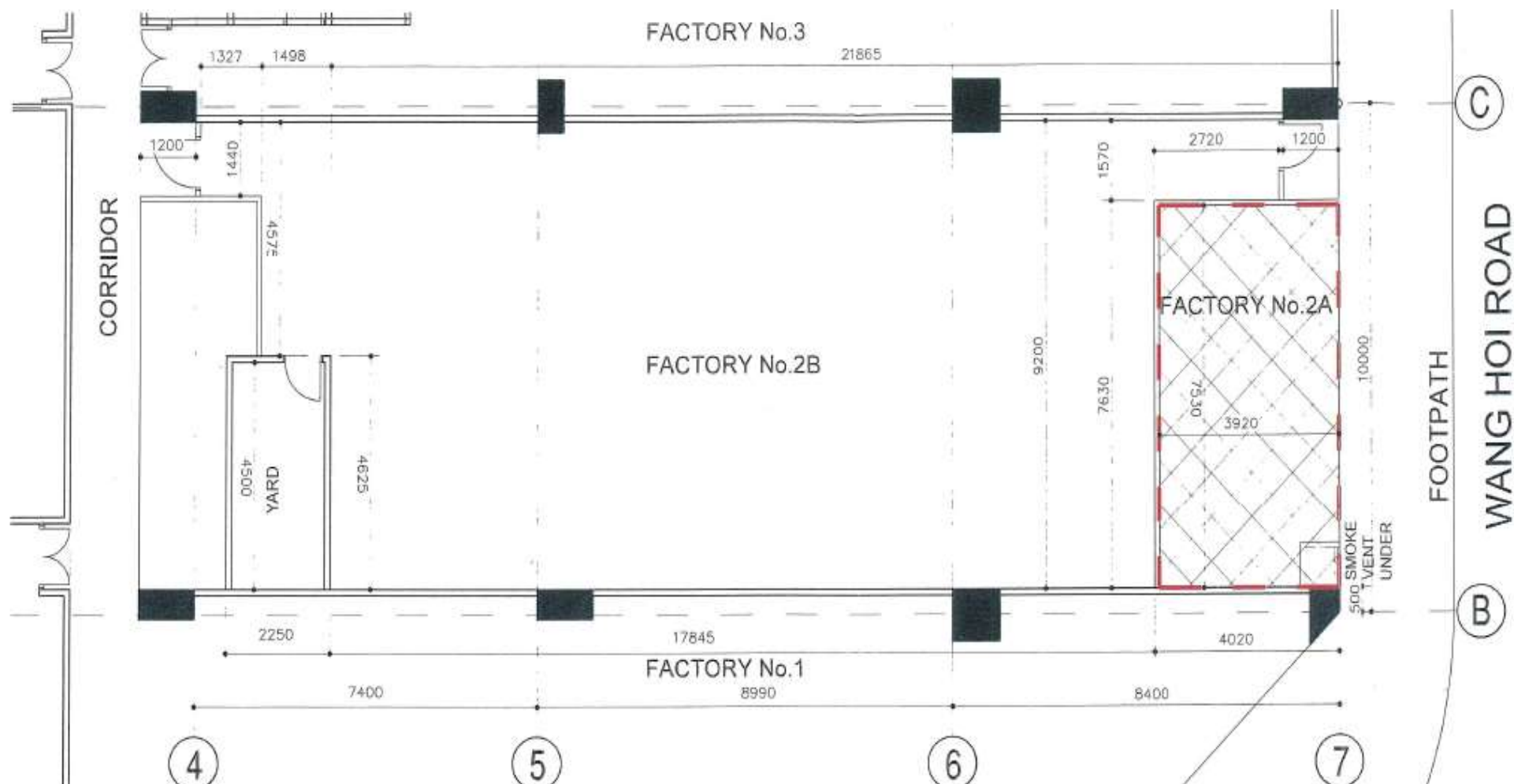
Unit Floor Plan 單位平面圖
