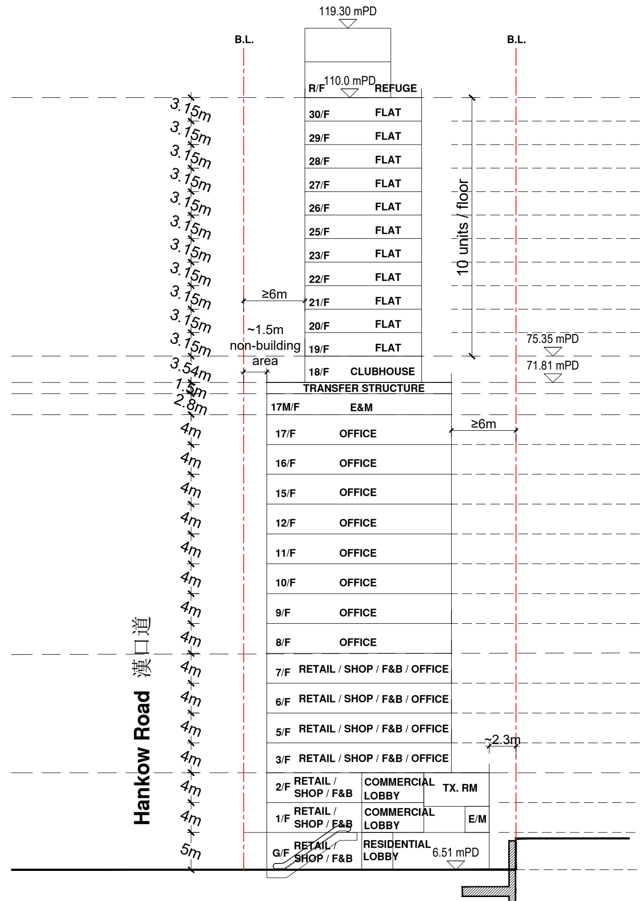
SECTION A-A
