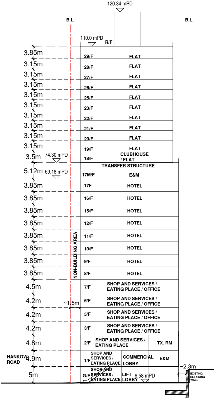
SECTION A-A
