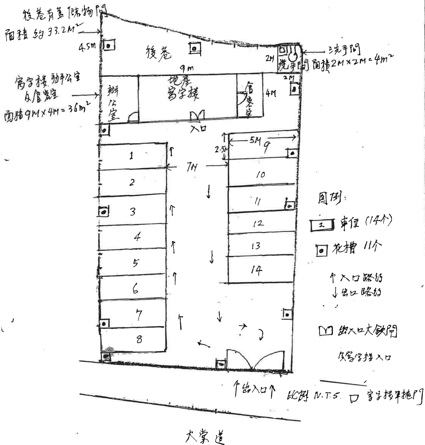
申請地點布局設計圖
