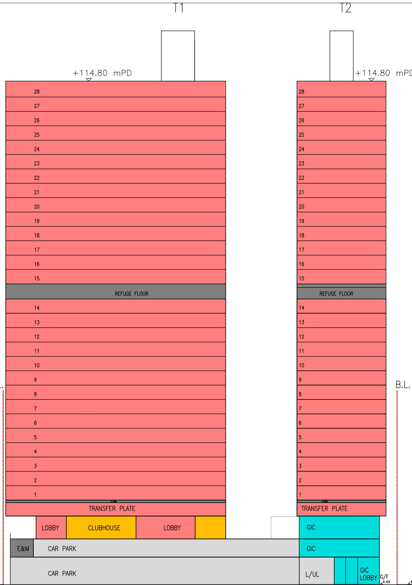
SECTION A-A
