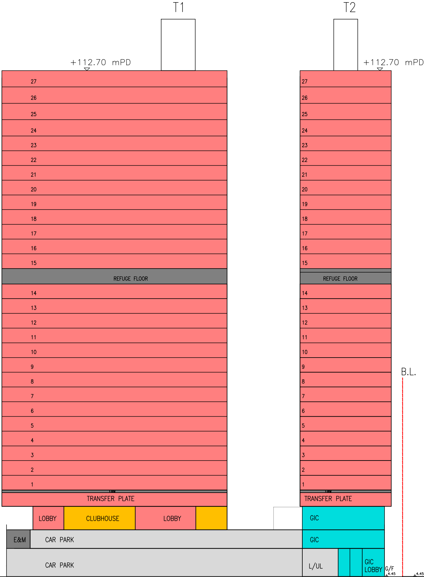
SECTION A-A
