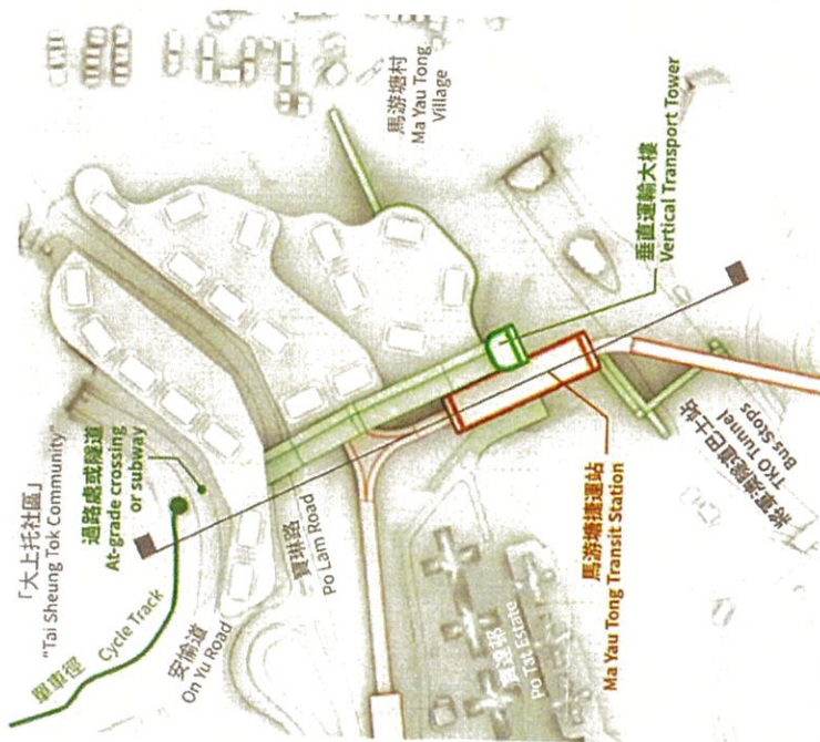
概念佈局 (非按比例) Concept layout (not to scale)
