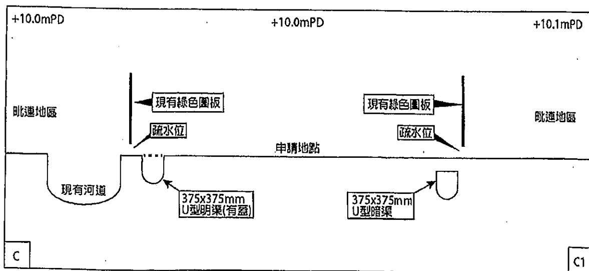
C—C1橫切面圖則
