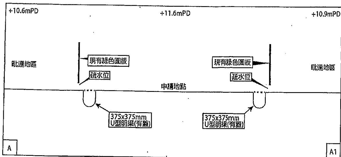
A—A1橫切面圖則
