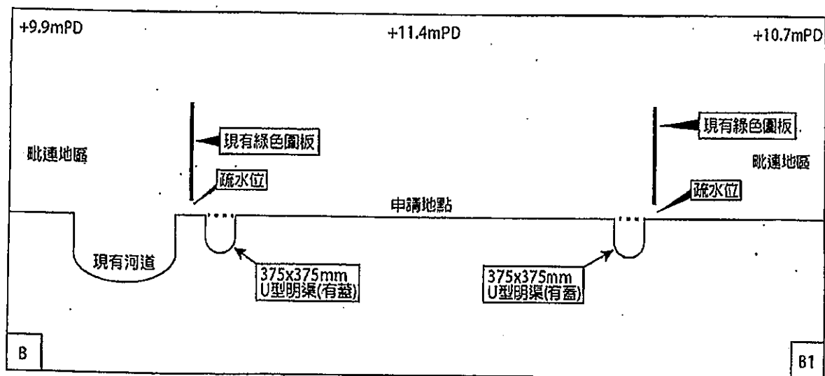
B—B1橫切面圖則
